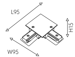
03 2202-CB-002 металл, пластик, IP20, 220V коннектор для линейного соединения треков под углом 90°
