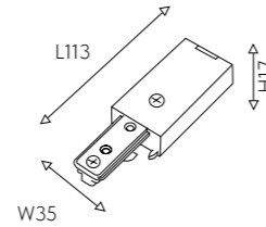
06 2201-BC-002 07 2201-WC-001 металл, пластик, IP20, 220V коннектор питания
