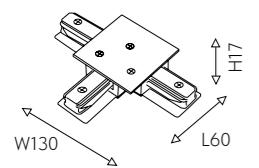
04 2202-CB-003 металл, пластик, IP20, 220V коннектор для Т-образного соединения треков
